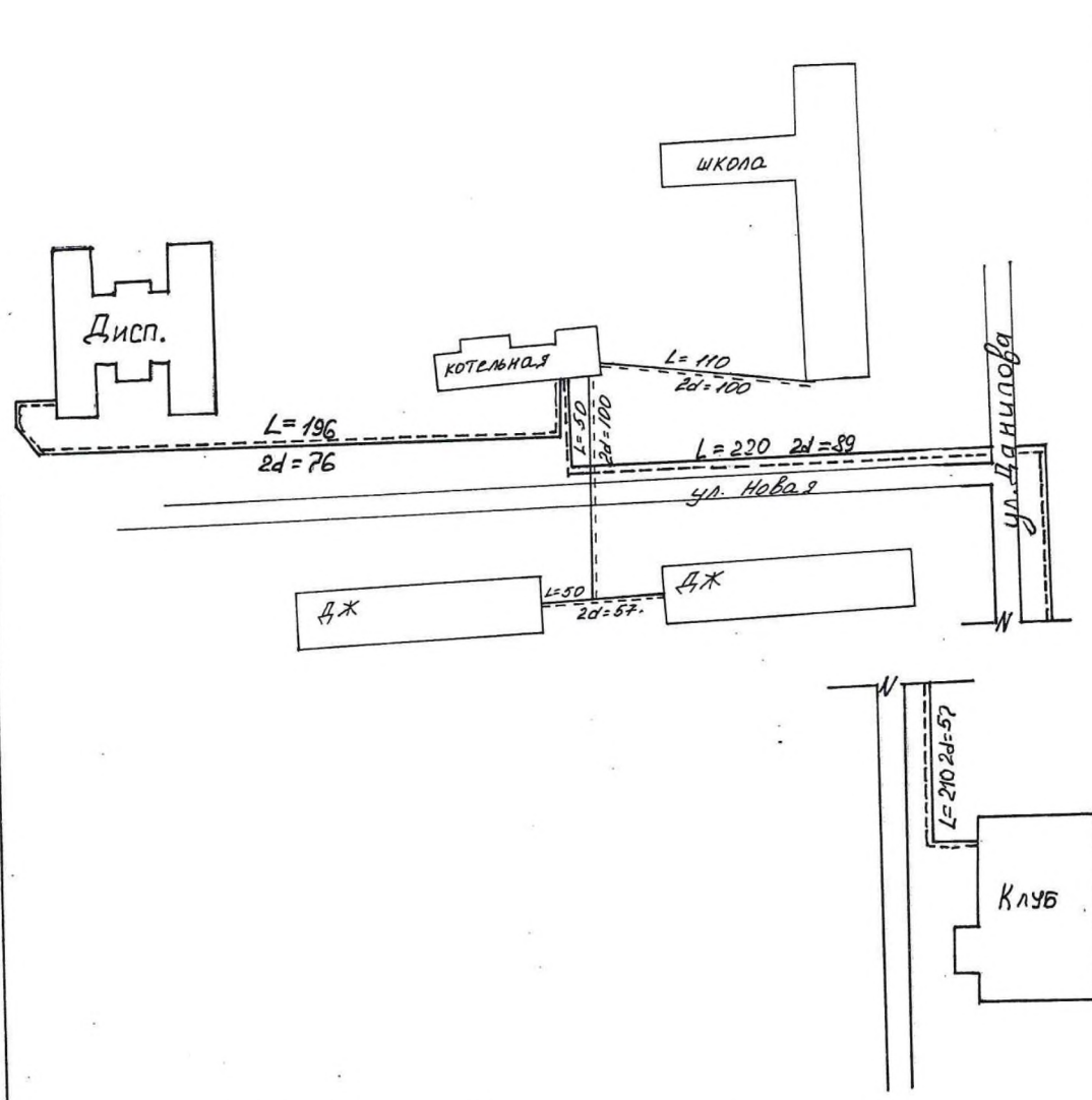
Рисунок 1.3.2.1 - Схема тепловой сети.
