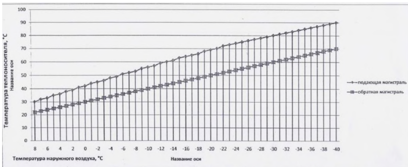
Рисунок 1.3.6.1 – Температурный график для котельных ООО «ЭНКОМ»
