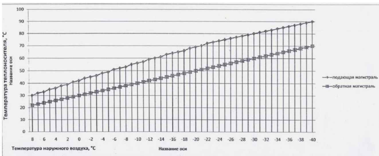
Рисунок 1.3.6.1 – Температурный график для котельных ООО «ТВР»
