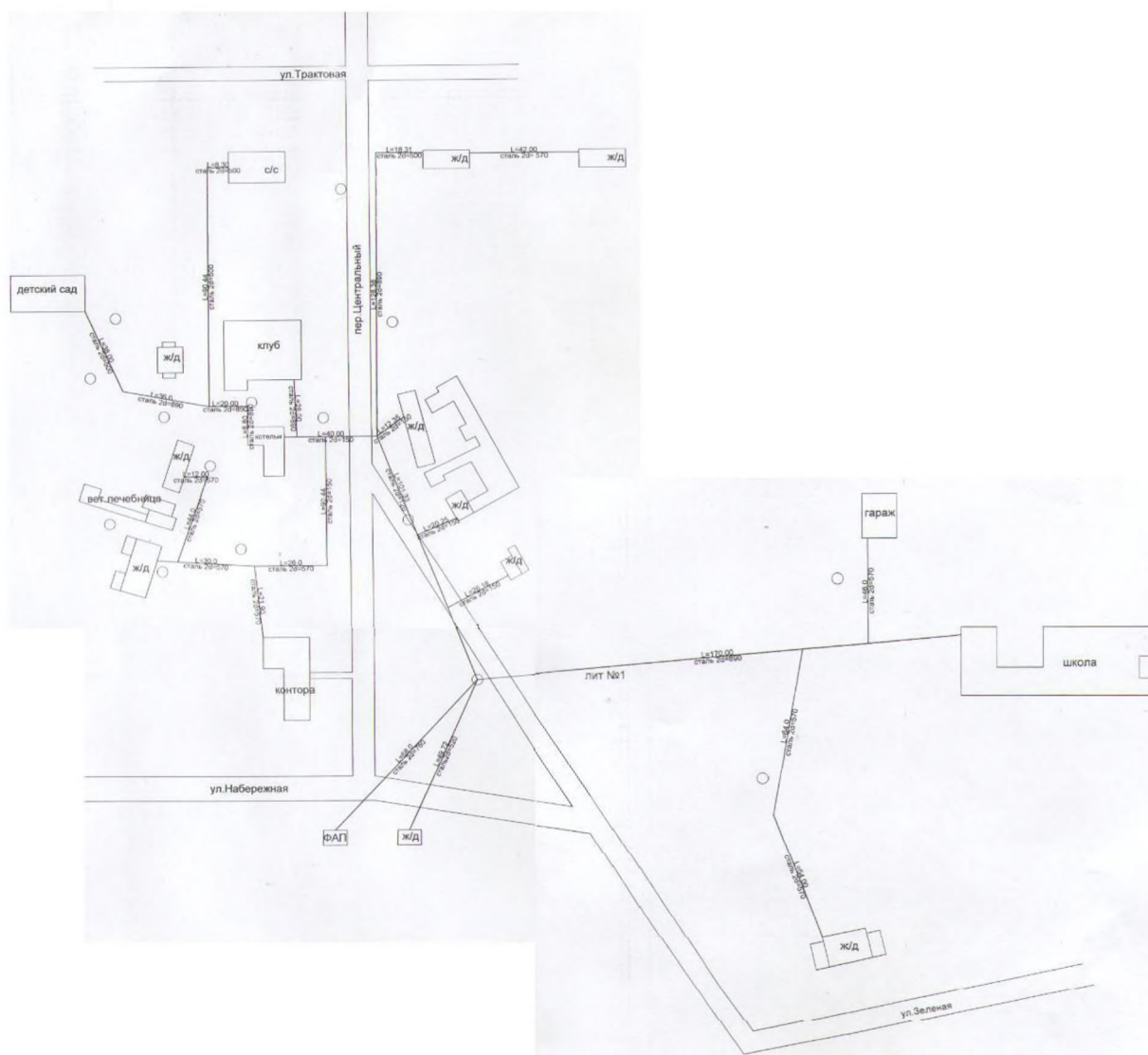
Рисунок 1.3.2.2 - Зона действия котельной, пер. Центральный, 4а
