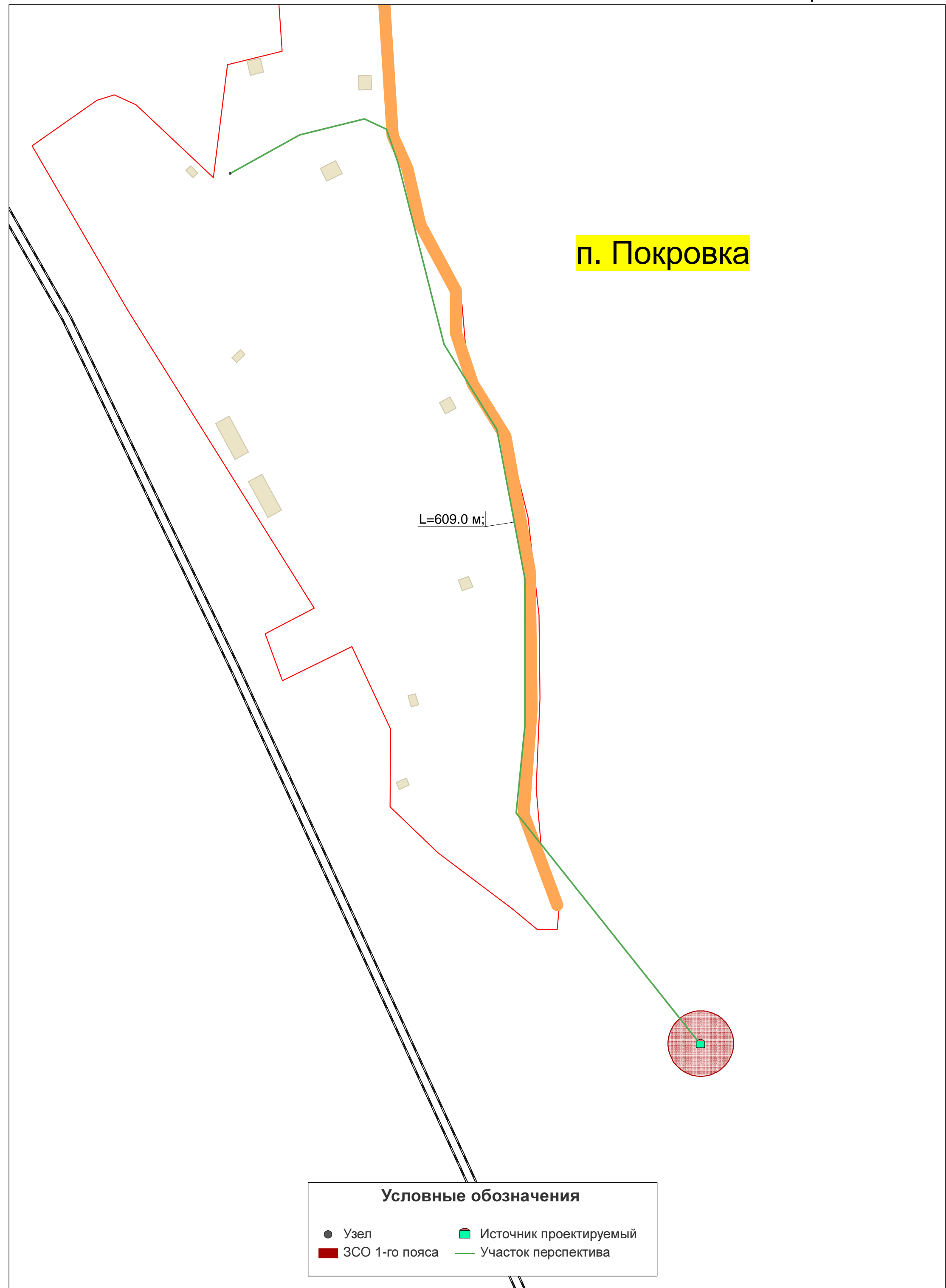
Рис. 5. Схема водоснабжения п. Покровка
