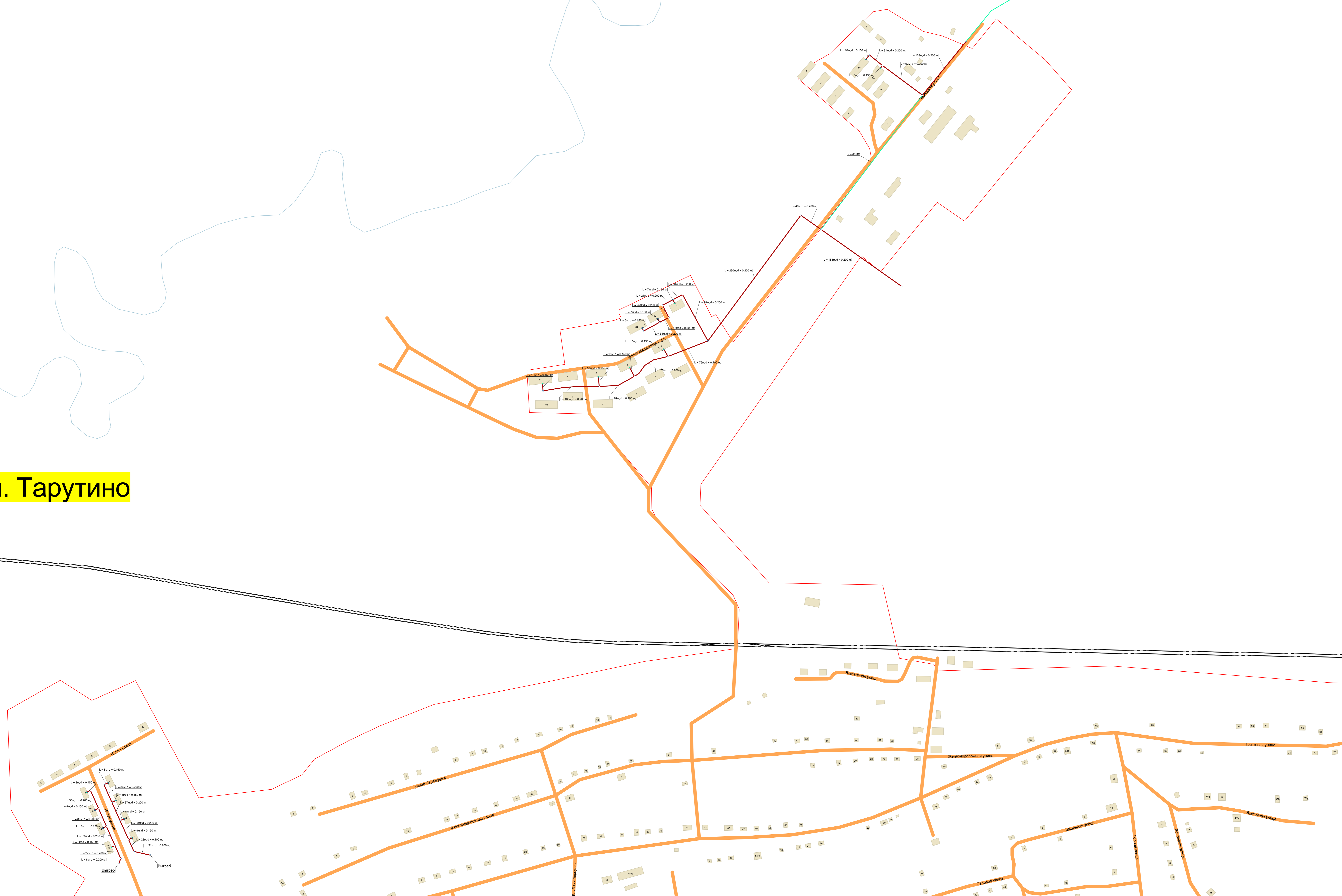
Рис.1. Схема водоотведения п. Тарутино
