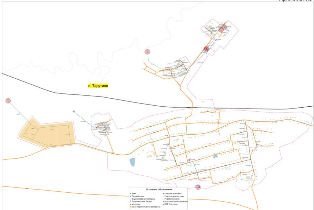
Рис.1. Схема водоснабжения п. Тарутино
