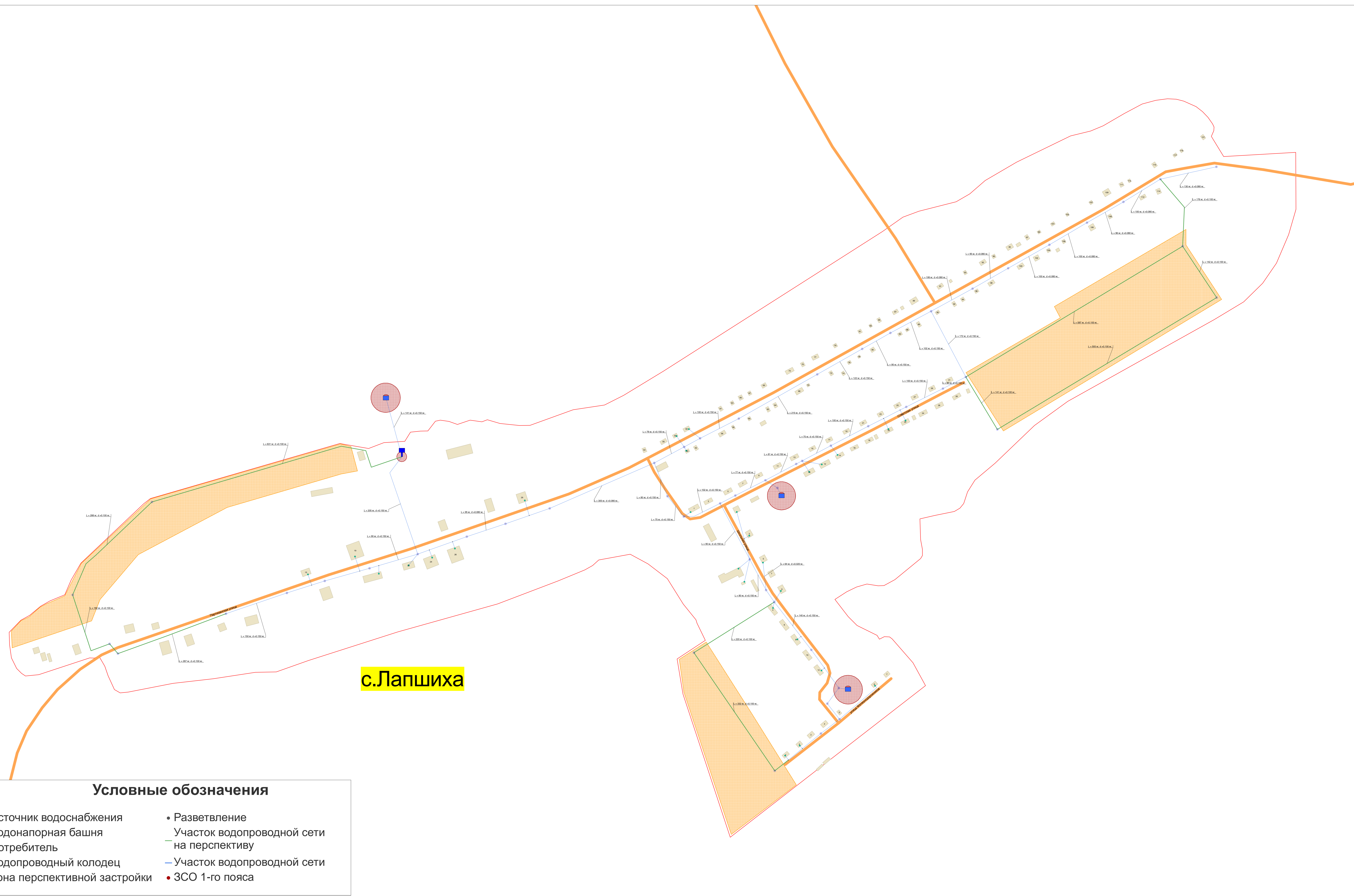
Рис. 1. Схема водоснабжения с.Лапшиха
