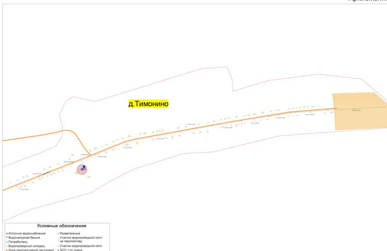
Рис. 2. Схема водоснабжения д.Тимонино
