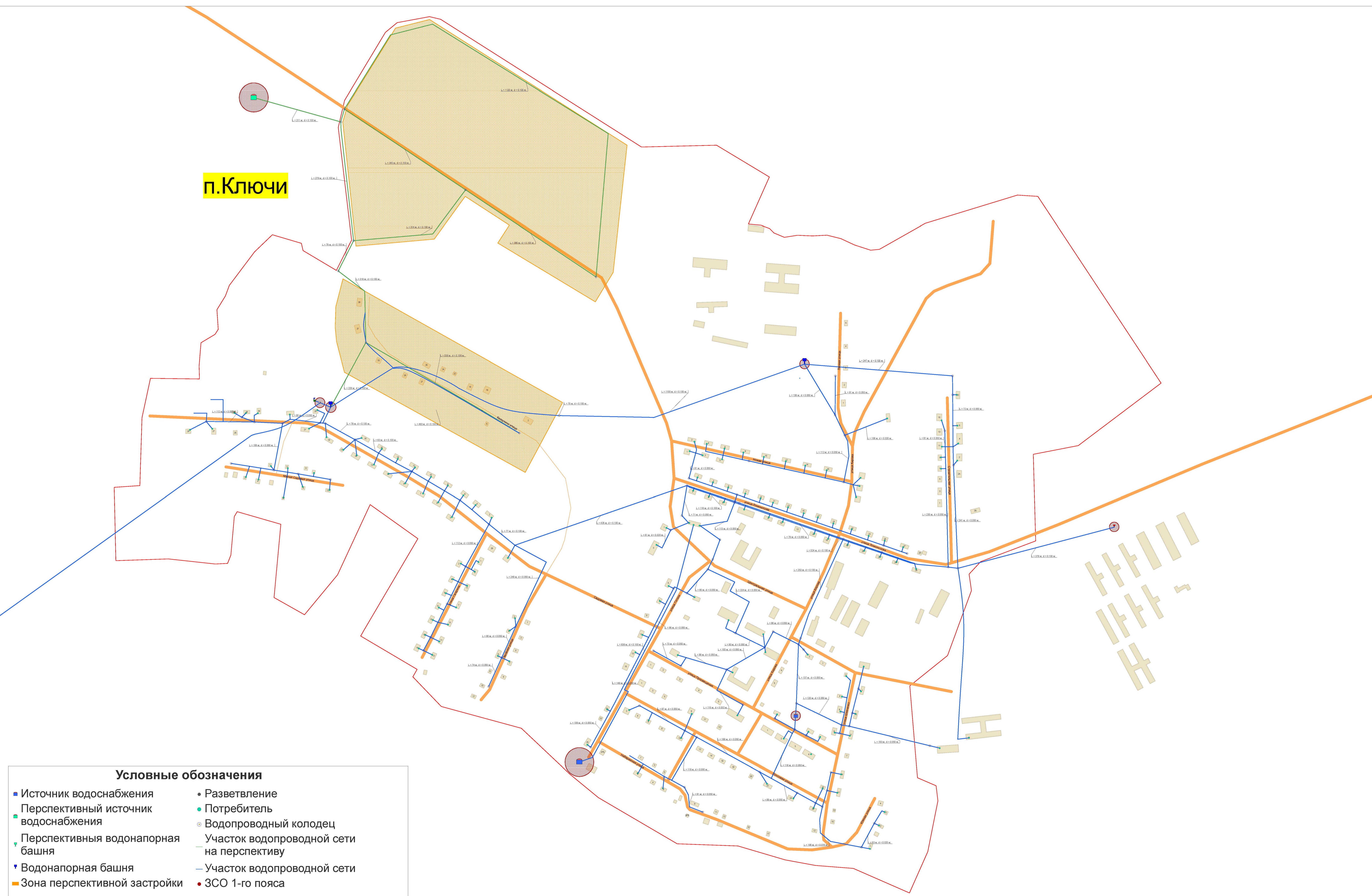
Рис. 1. Схема водоснабжения п.Ключи
