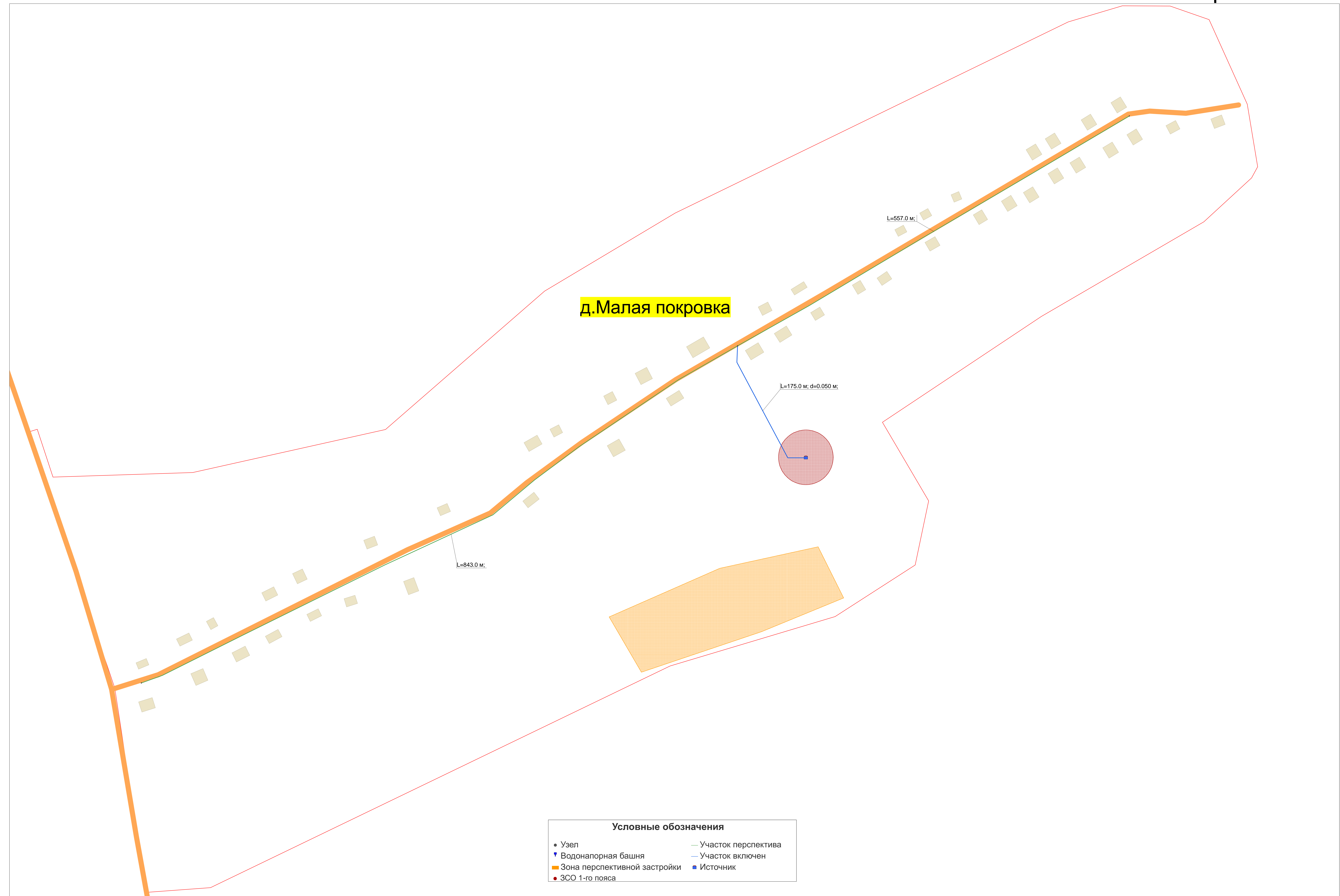
Рис. 4. Схема водоснабжения д. Малая Покровка
