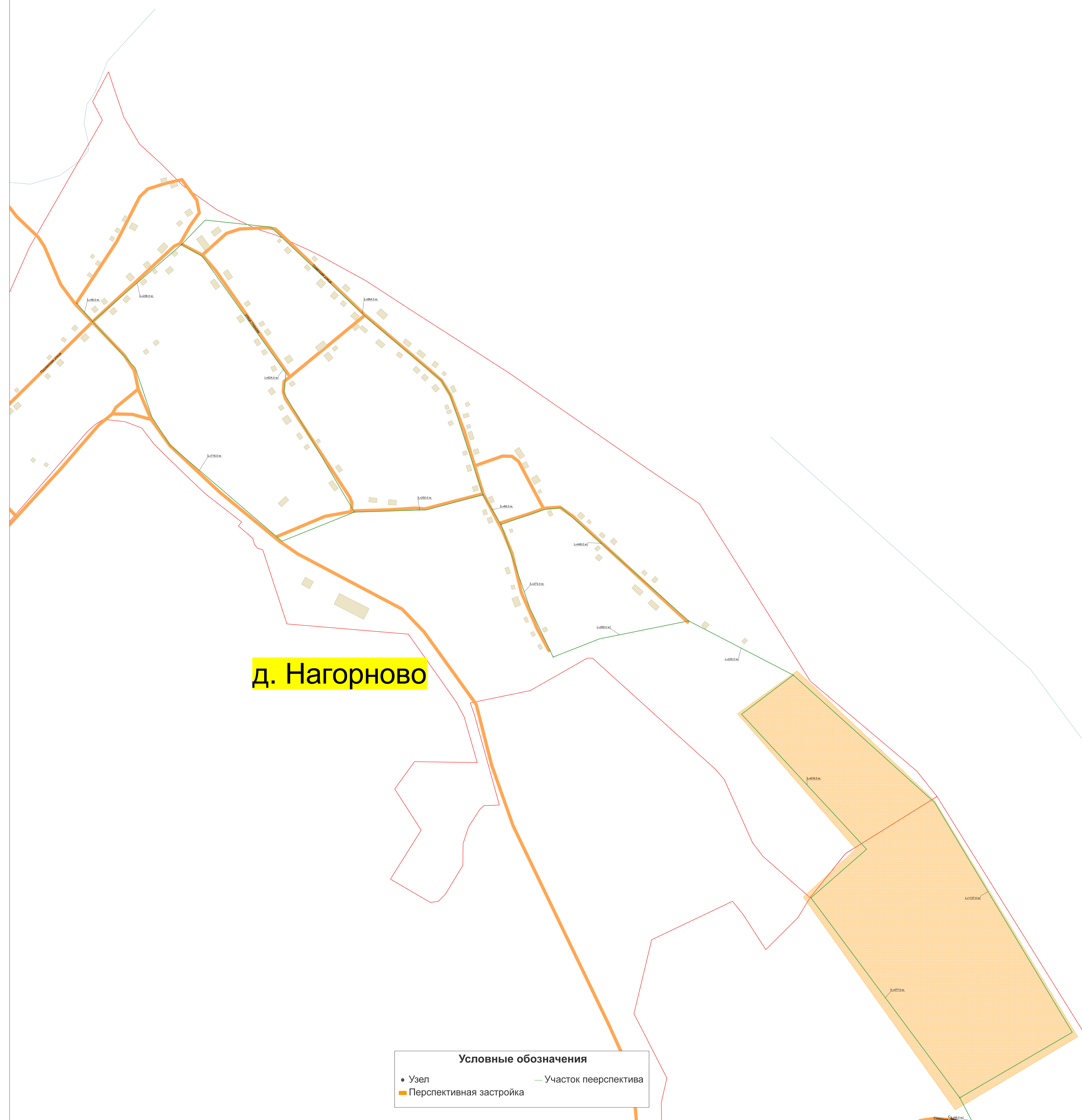
Рис. 2. Схема водоснабжения д. Нагорново
