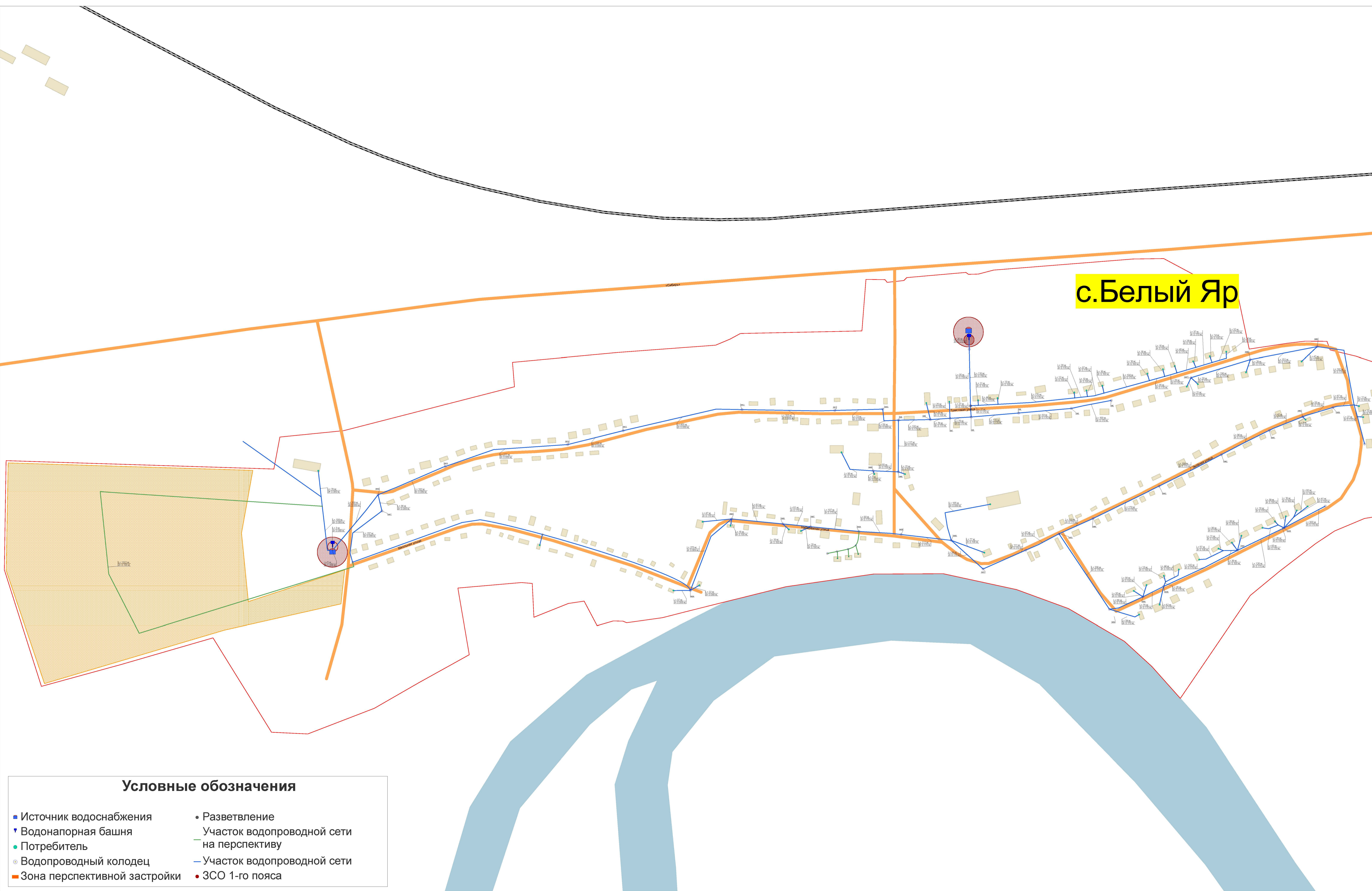
Рис. 1. Схема водоснабжения с.Белый Яр
